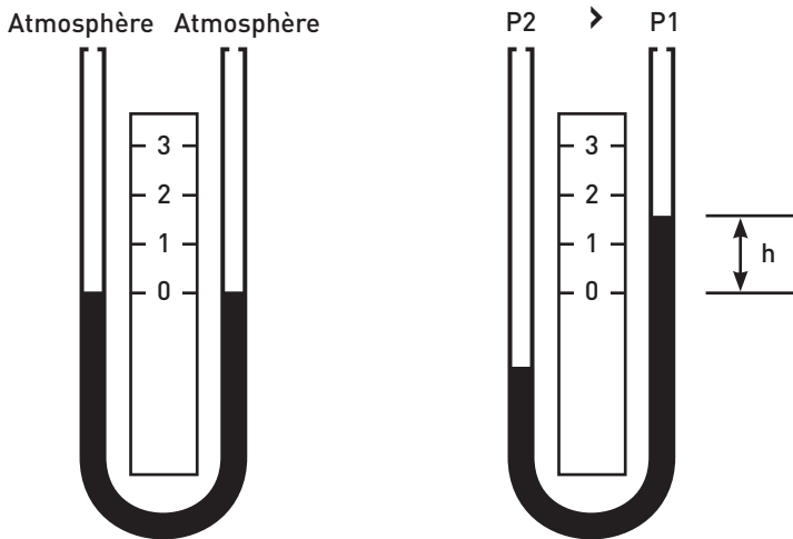
Figure 7 ↑ Manomètre à tube en U.
